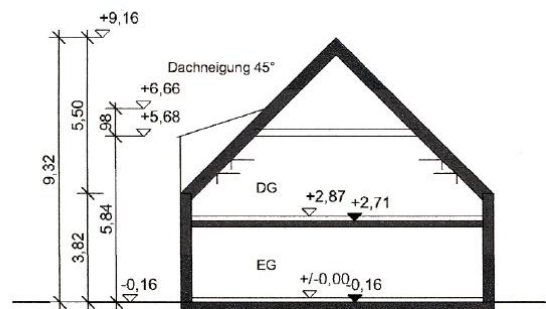
SYSTEMSCHNITT HAUS 2
