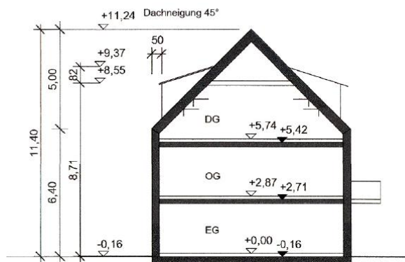
SYSTEMSCHNITT HAUS 1
